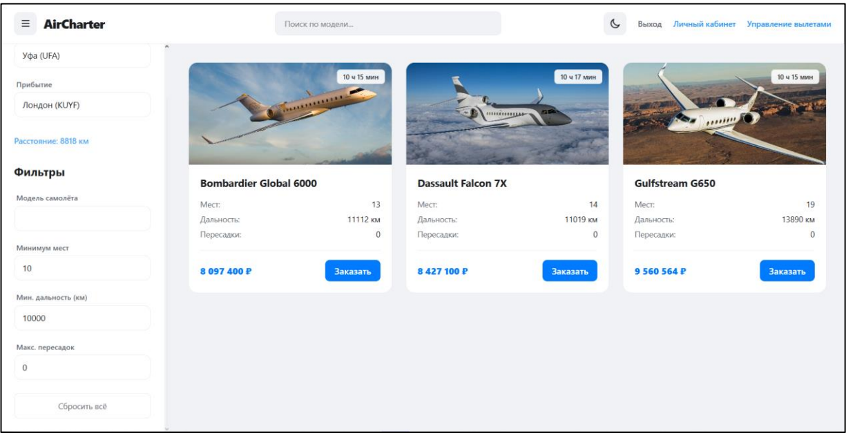
Рисунок 2.3.8 – Фильтрация каталога
